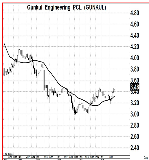
Price Chart...(GUNKUL)
